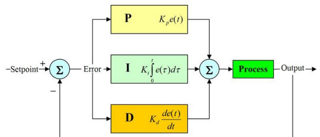
Fig. 3 PID BLOCK
